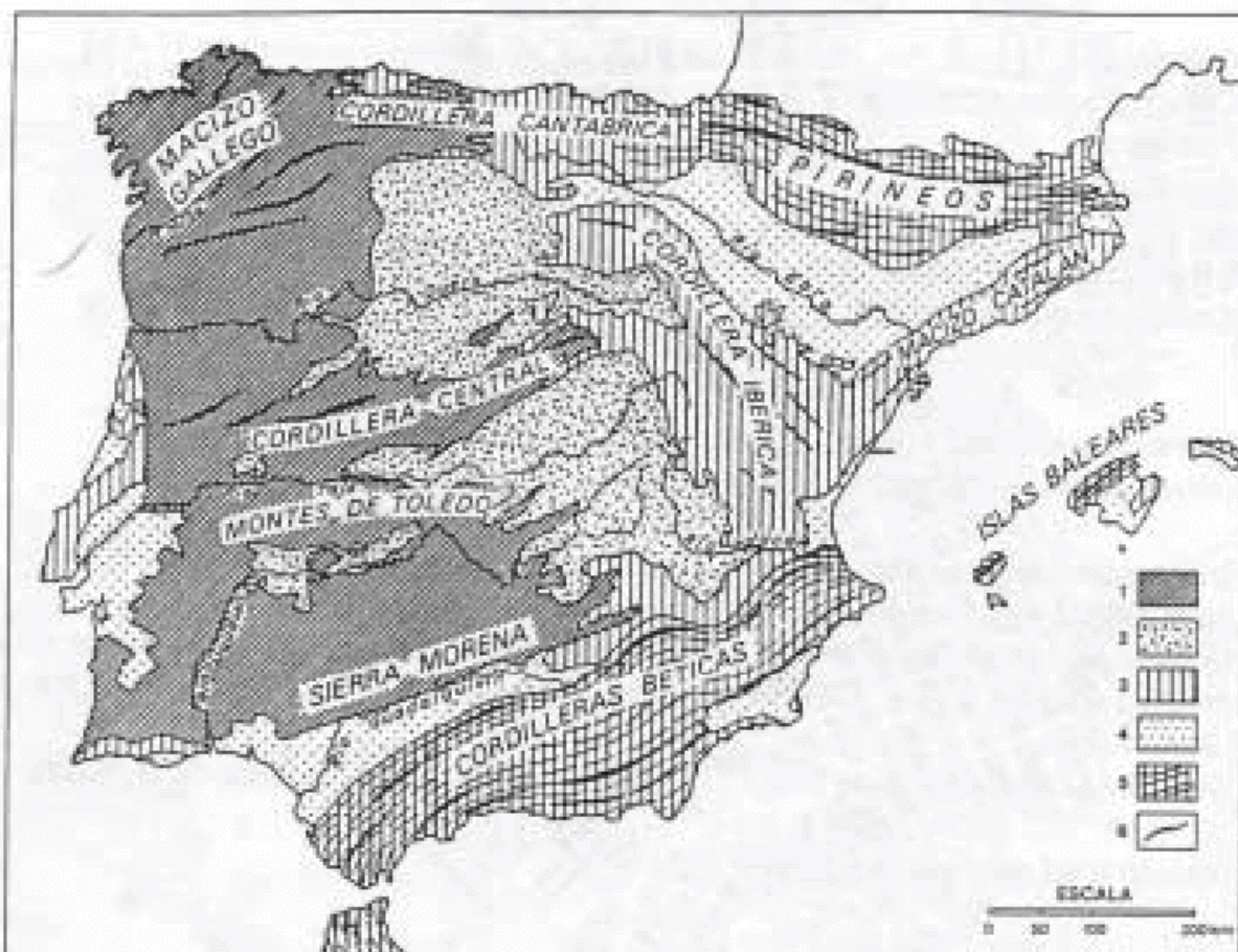
FIG. 4. — Grandes conjuntos estructurales de la Península Ibérica. Signos convencionales: 1) Macizo hercínico de la Meseta o bloque hespérico; 2) Depresiones tectónicas de la Meseta; 3) Rebordes alpinos de la Meseta; 4) Depresiones periféricas; 5) Cordilleras alpinas; 6) Direcciones de las principales alineaciones montañosas.
